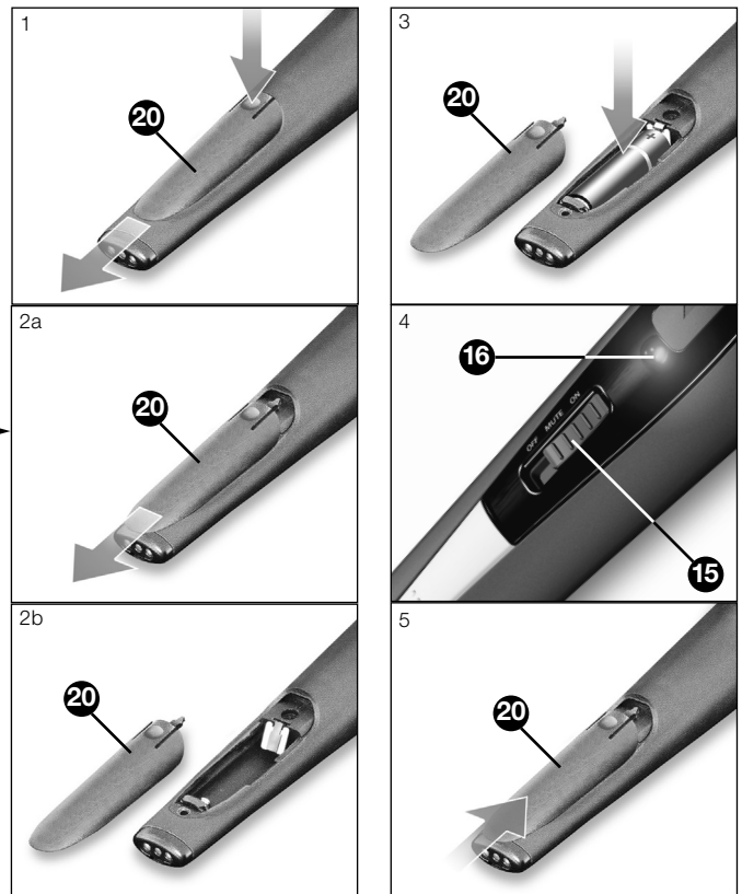
Fig. 8 / HT 40 FLEXX
