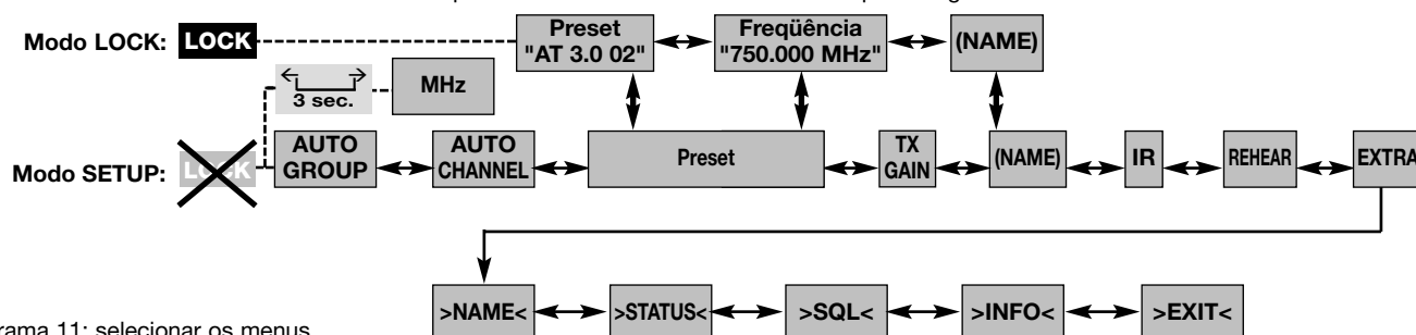
Diagrama 11: seleccionar os menus
