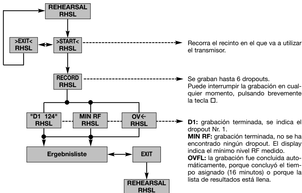
Diagrama 9: Función Rehearsal
