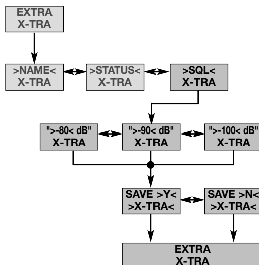
Diagramme 10 : réglage du seuil d'atténuation.
