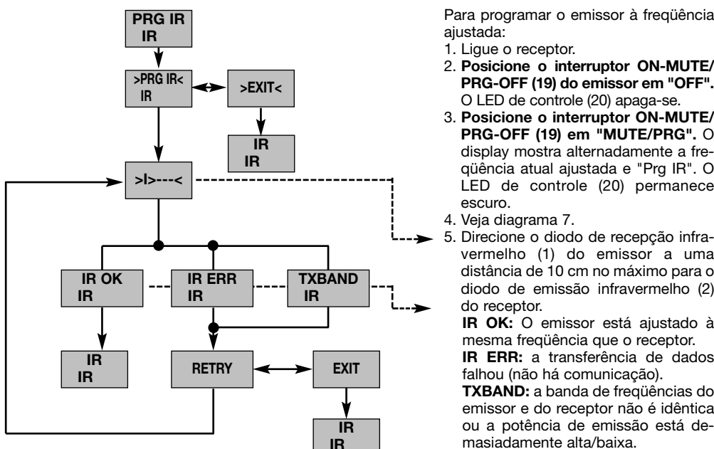
Diagrama 7: ajustar a frequência portadora do emissor
