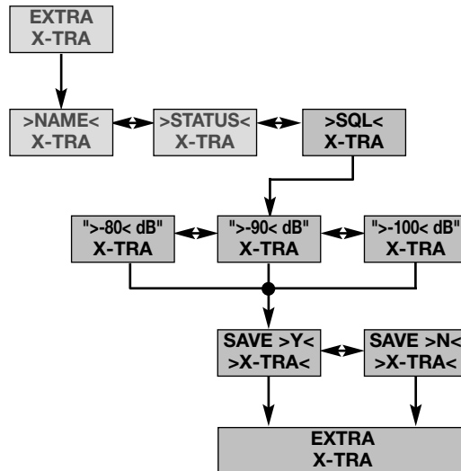
Diagrama 10: Ajustar el nivel silenciador
