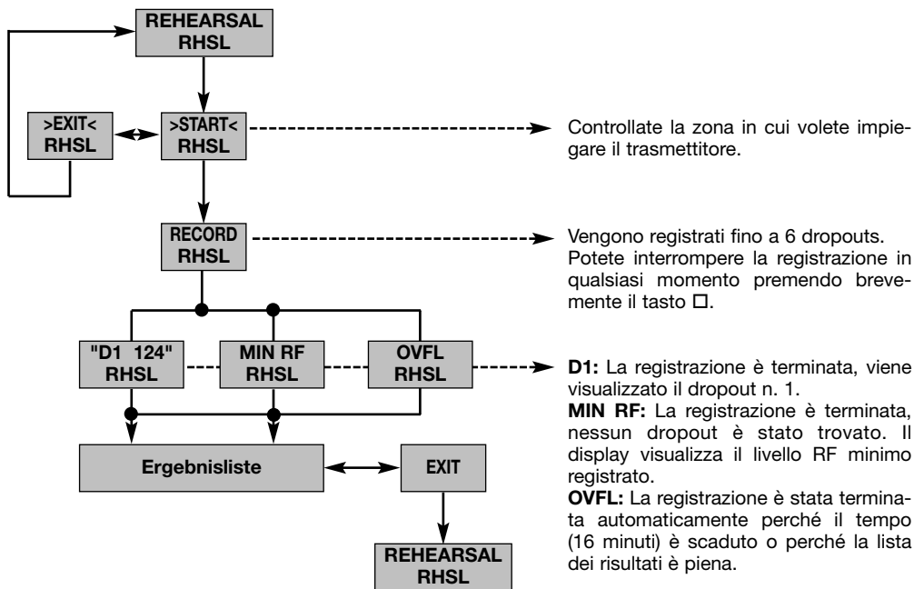
Diagramma 9: Funzione Rehearsal
