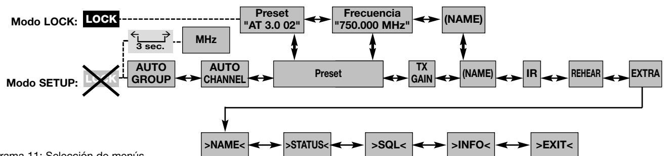
Diagrama 11: Selección de menús
