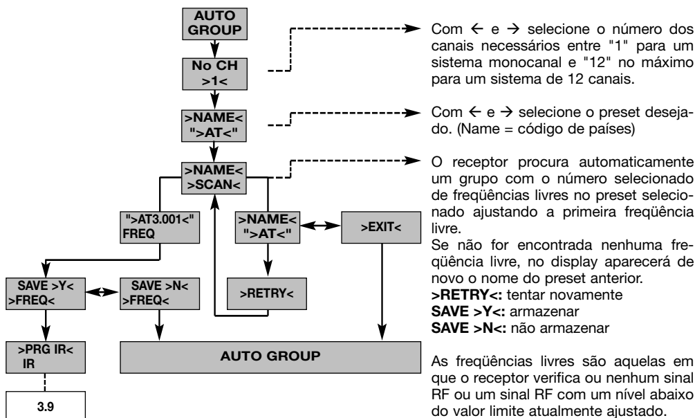
Diagrama 3: procura automática de um grupo de freqüências livres.
