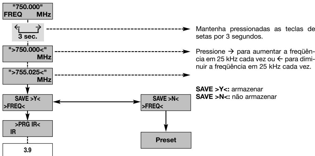
Diagrama 5a: ajustar a frequência diretamente.
