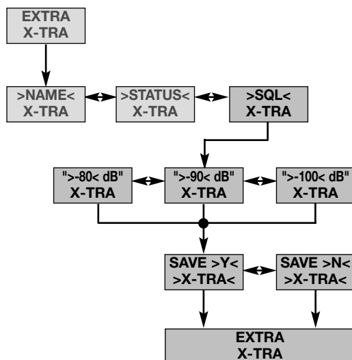
Diagrama 10: ajustar o nível do squelch.
