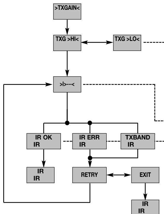
Diagrama 8: ajustar a sensibilidade de entrada do emissor de mão
