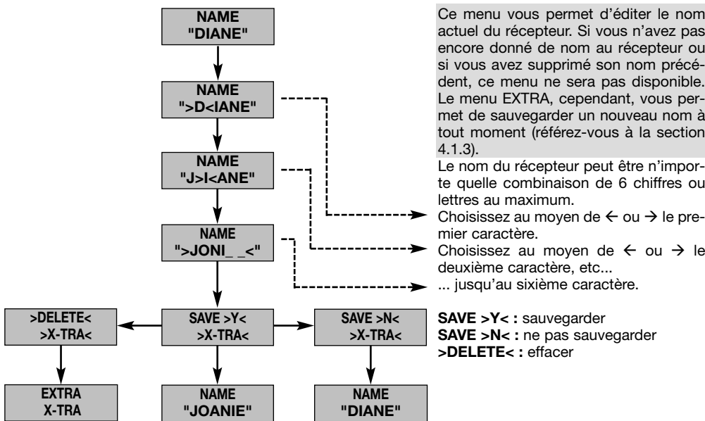
Diagramme 6 : modification du nom attribué au récepteur
