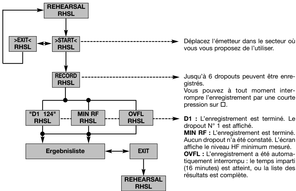
Diagramme 9 : Fonction de répétition
