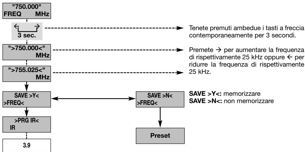
Diagramma 5a: Come regolare la frequenza direttamente.
