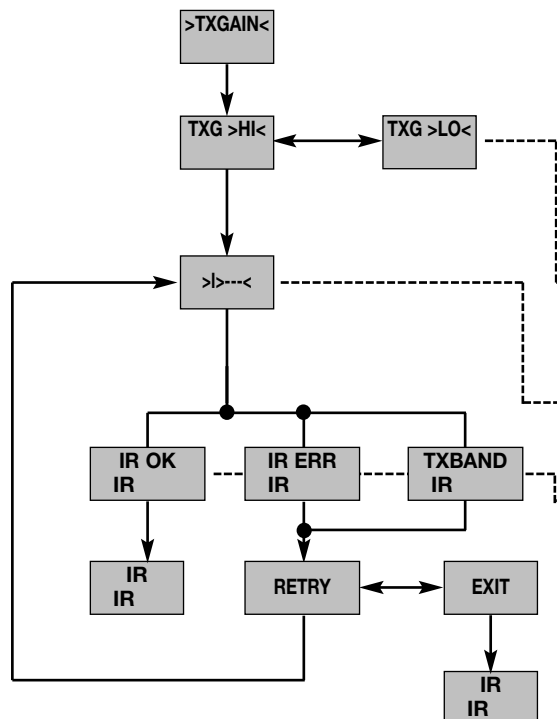
Diagramme 8 : réglage de la sensibilité d'entrée de l'émetteur à main
