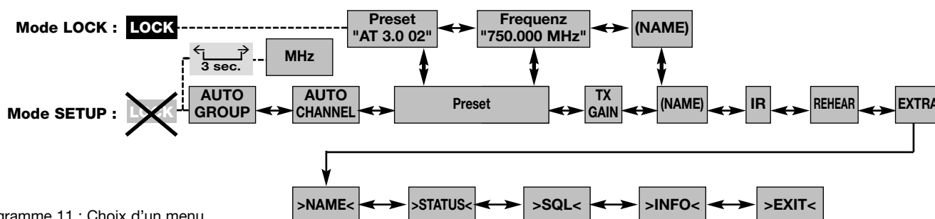
Diagramme 11 : Choix d'un menu
