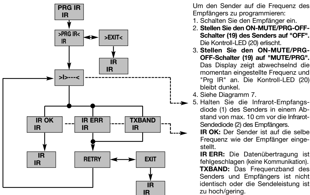
Diagramm 7: Trägerfrequenz des Senders einstellen
