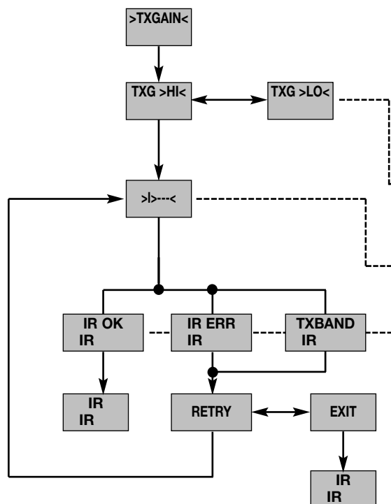
Diagrama 8: Ajustar la sensibilidad de entrada del transmisor manual
