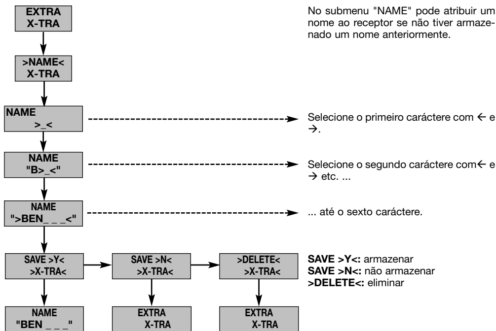
Diagrama 12: introduzir novos nomes para o receptor
