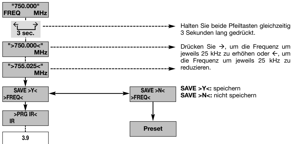
Diagramm 5a: Frequenz direkt einstellen.
