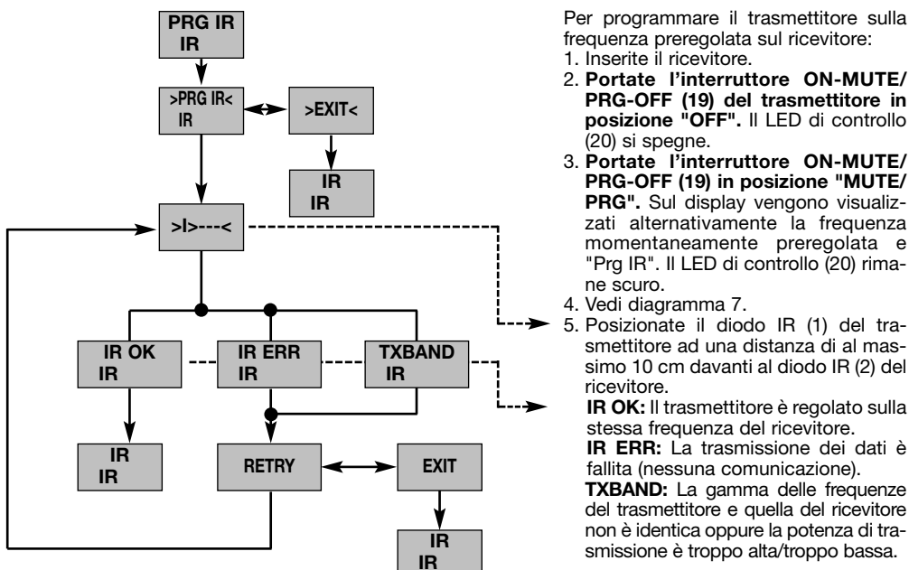
Diagramma 7: Come regolare la frequenza portante del trasmettitore
