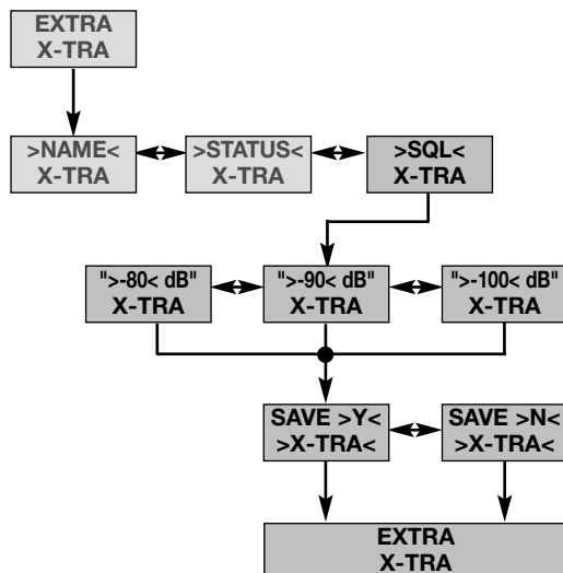
Diagramm 10: Squelchpegel einstellen.
