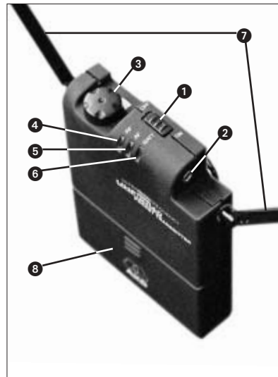
Abb. 1: Bedienelemente (Oberseite)
