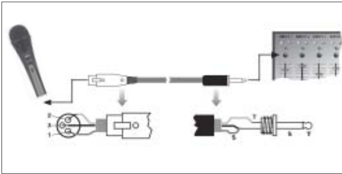
Fig. 5: Collegamento tramite cavo asimmetrico
