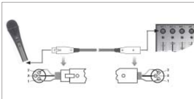
Fig. 4: Collegamento tramite cavo XLR simmetrico
