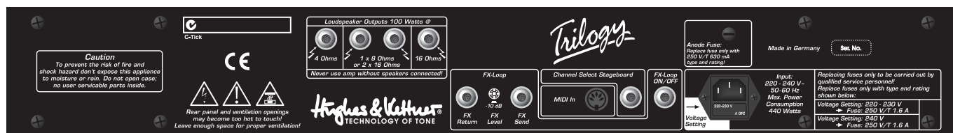
Abb. 2: Trilogy Rückseite
