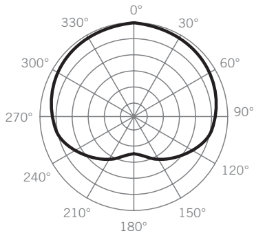
Patrón polar
