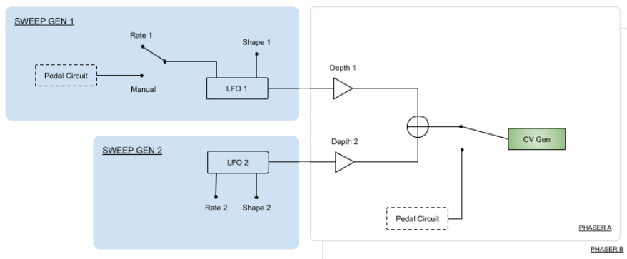
Diagrama de flujo de la señal del pedal
