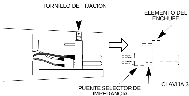
SELECCION DE IMPEDANCIA - EXTREMO DEL RECEPTACULO DEL MICROFONO
