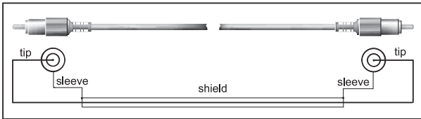
Fig. 4.4: RCA cable
