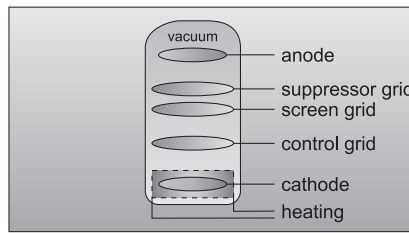
Fig. 1.5: pentode
