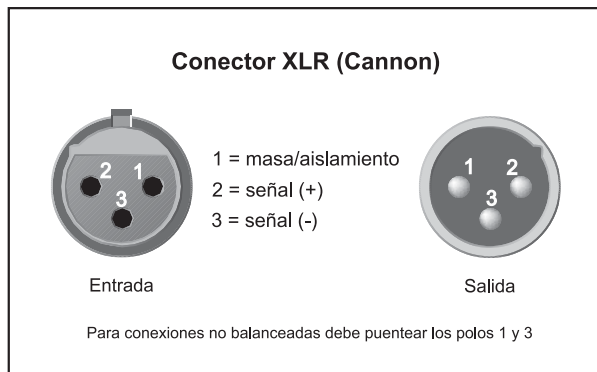
Fig. 4.1: Conexiones XLR
