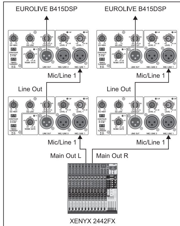
Fig. 3.3: Conexión en serie de varios B415DSP
