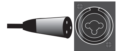
Entrée Microphone sur Prise Combo XLR/Jack 6.35mm (3)
