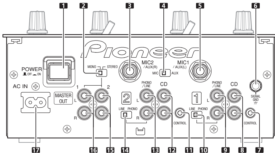
Panneau arrière
